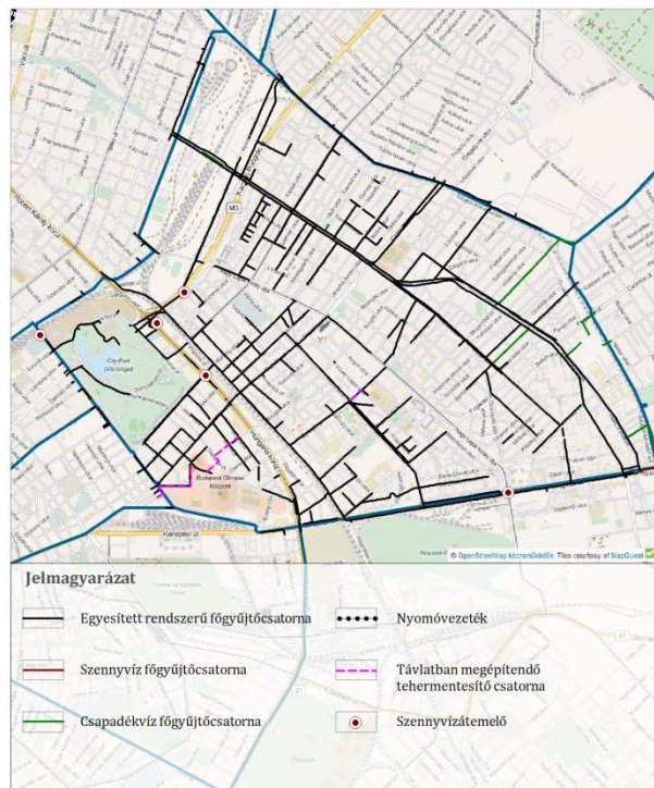
102. ábra: Csatorna főgyűjtő hálózat
