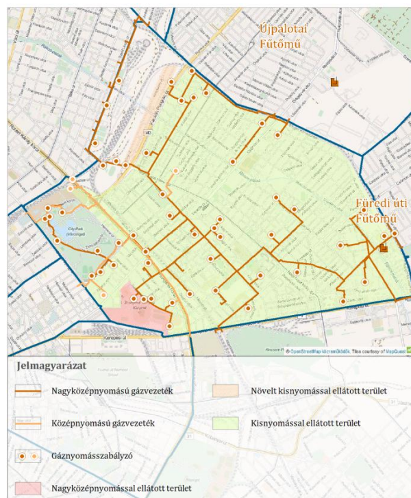
106. ábra: Gázellátás
