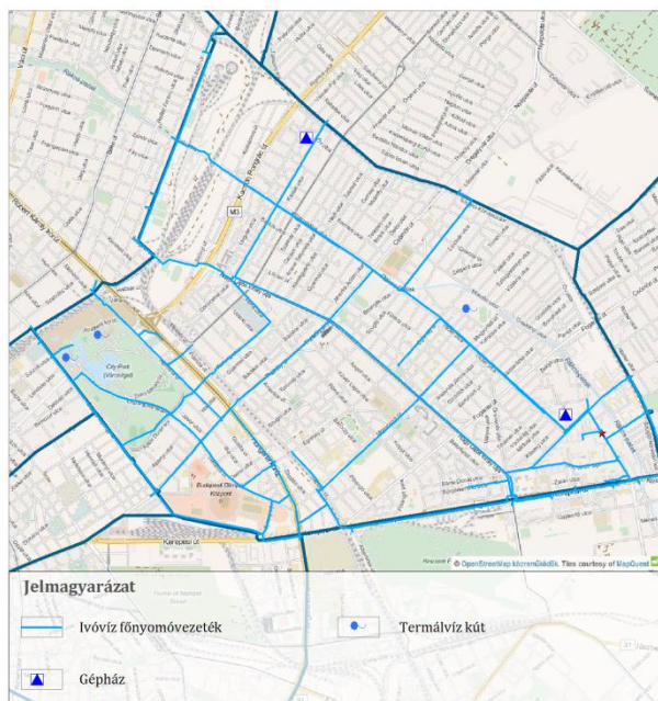
101. ábra: Ivóvíz főnyomó vezetékek
