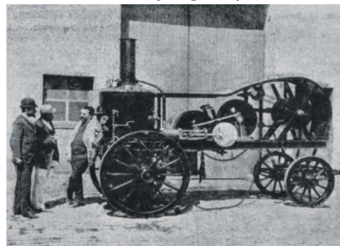
Ilyen volt a huszonöt lóerős gőzgép, amely a léggömb emelkedését szabályozta
