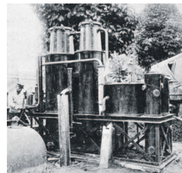
A hidrogént a helyszínen állították elő vasforgácsra öntött kénsav és víz keverékéből
